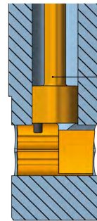
블레이드가 접힌 블레이드 하우징
