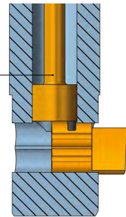
블레이드가 확장된 블레이드 하우징 - 로커가 피니언의 회전 운동을 통해 블레이드를 바깥쪽으로 이동시킵니다.
